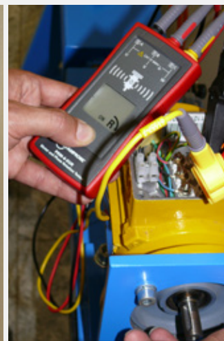
Spannungsfreie Ermittlung der Motoranschlüsse vor der Inbetriebnahme
