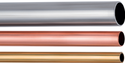
Zum Schneiden von Kupfer-, Messing- und Edelstahlrohren mit einer Wandstärke bis 2 mm und einem Durchmesser von 6 - 35 mm (1/4" - 1 3/8")
