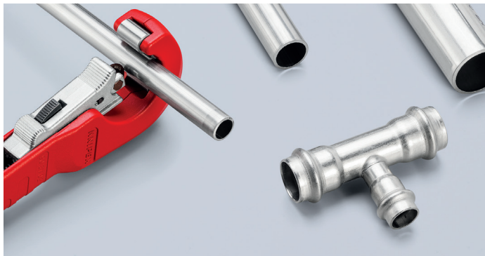
Schneller im Arbeitsalltag: Dank QuickLock-Einhandschnellverstellung rutscht das Schneidrad mit einem einzigen Daumendruck an jeden Rohrdurchmesser heran
