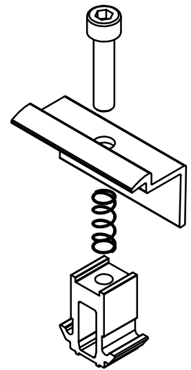
Isometrie 1 : 2
