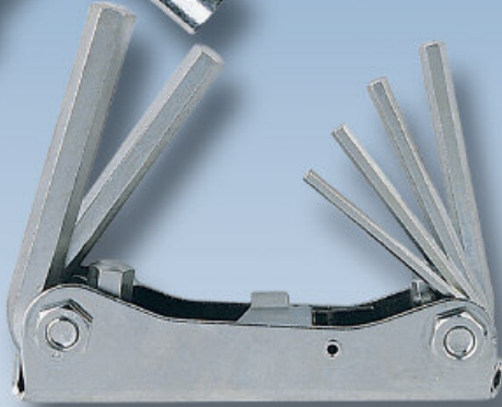
Universal- Sechskant- Stiftschlüssel
