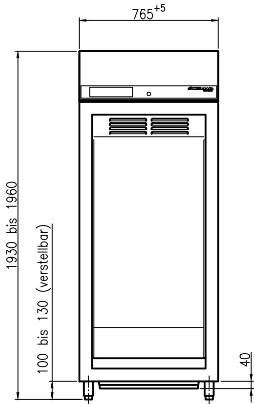
Ansicht ohne Türe gezeichnet
