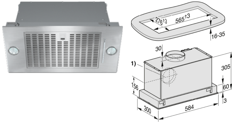
DA 2360 (Skizze)
