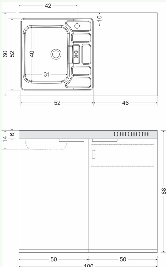
Skizze / Maße
