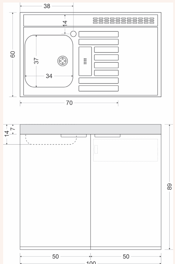
Skizze / Maße
