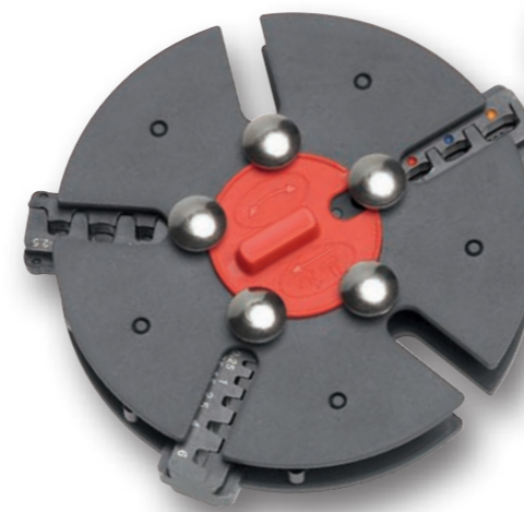
97 33 01 Crimpzange mit Rundmagazin und 3 Wechselseinsätzen für unisolierte, offene Steckverbinder; isolierte Kabelschuhe + Steckverbinder; Aderendhülsen
