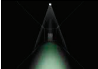
Micropoint 2 E AT Fluchtwegausleuchtung mit asymmetrischer Optik
