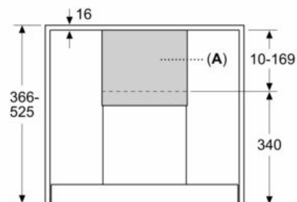
Maße in mm Einbaubeispiel für Schrankhöhe 366-525 mm
