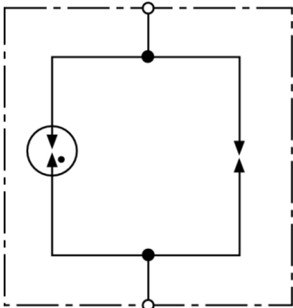
Prinzipschaltbild SDS 2
