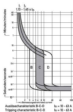
Diagramme Leitungsschutzschalter DLS 6h B32-3+N
