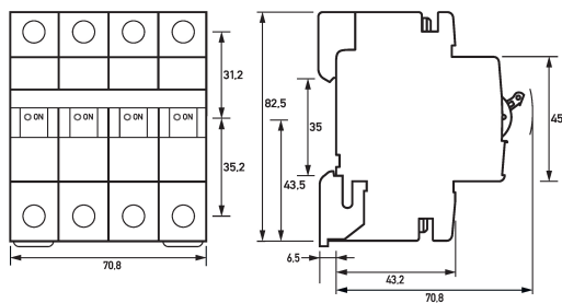
Maßzeichnung Leitungsschutzschalter DLS 6h B32-3+N
