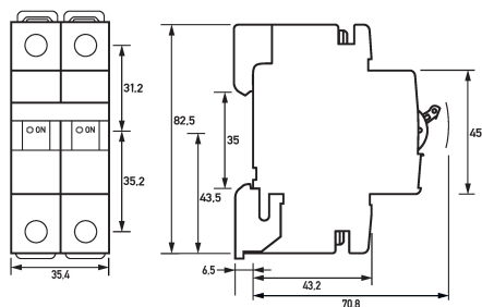
Maßzeichnung Leitungsschutzschalter DLS 6i Bo4-1+N
