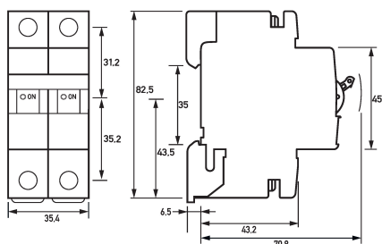
Maßzeichnung Leitungsschutzschalter DLS 6h C6-2
