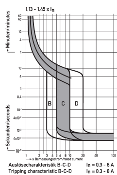
Diagramme Leitungsschutzschalter DLS 6h C6-2
