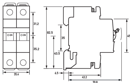
Maßzeichnung Leitungsschutzschalter DLS 6i Bo4-2
