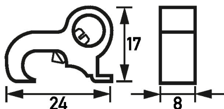
Maßzeichnung Wiedereinschalt sperren RH-SPE
