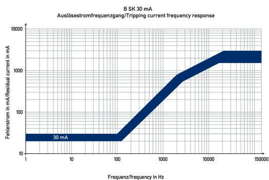
Diagramme Fehlerstromschutzschalter DFS 4 063-4/0,03-B SK NA R
