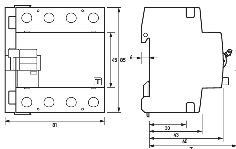
Mazeichnung Fehlerstromschutzschalter DFS 4 063-4/0,03-B SK NA R
