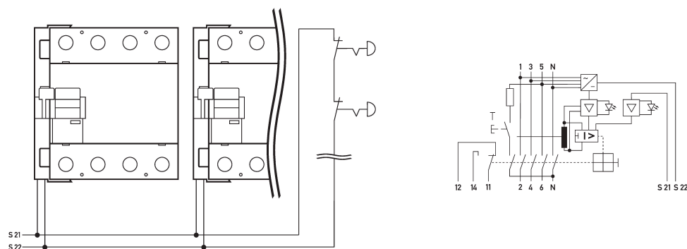
Schaltungsbeispiel Fehlerstromschutzschalter DFS 4 063-4/0,03-B SK NA R
