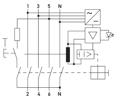
Schaltungsbeispiel Fehlerstromschutzschalter DFS 4 063-4/0,10-PV R HD
