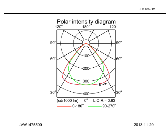
IFPC1_TCS640 3xTL5-14W HFP AC-MLO.EPS
