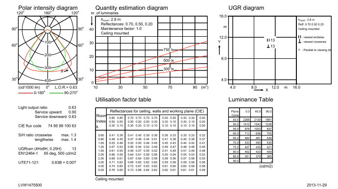
TCS640 3xTL5-14W HFP AC-MLO
