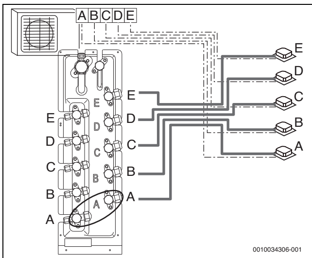
Bild 18 Übersicht Anschlussklemmen
