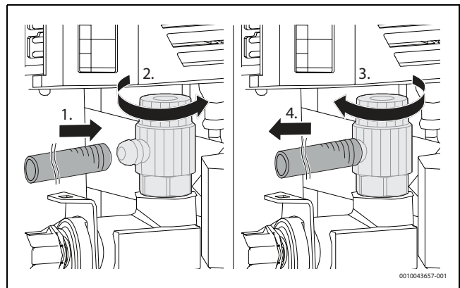
Bild 23 Entlüfter öffnen und schließen am Beispiel des Entlüfters an der Primärkreispumpe
