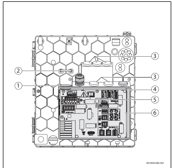
Bild 32 Kabelführung im Anschlussbereich für Netzkabel
