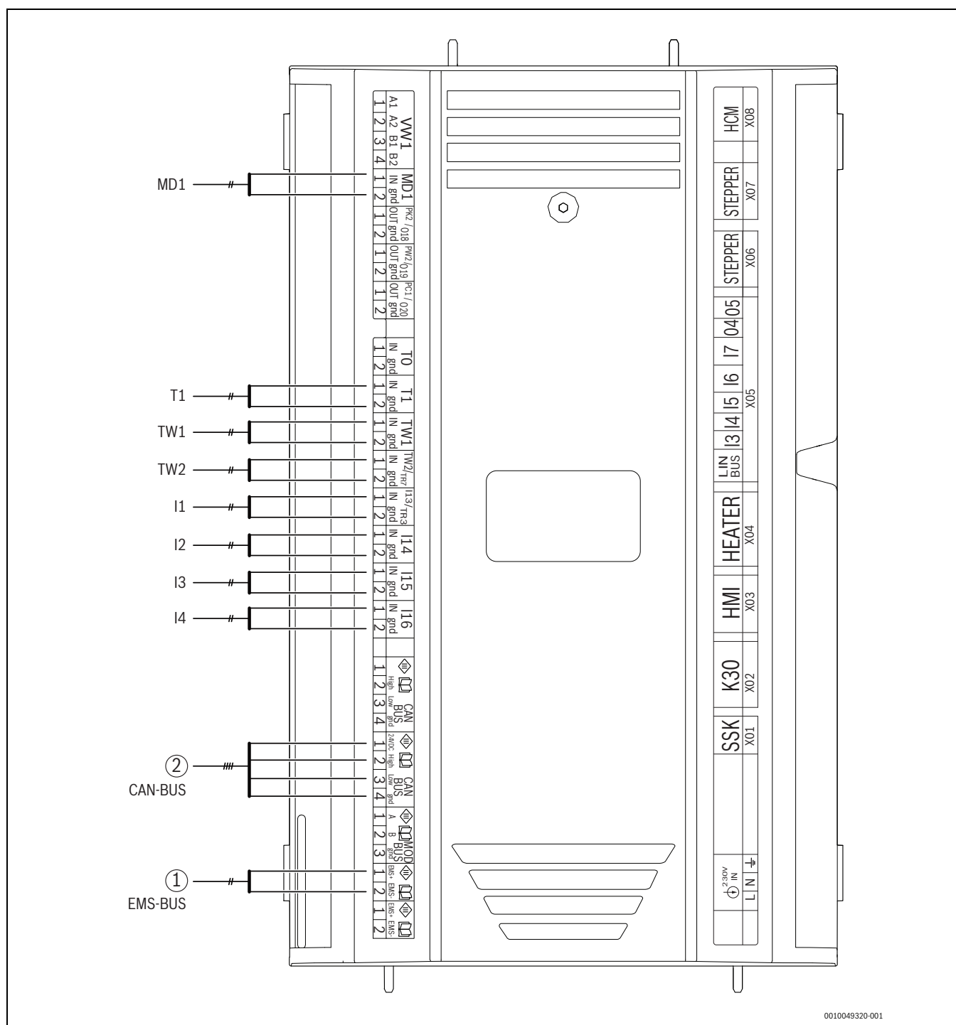
[MD1] Kondensationsfühler (Zubehör für Kühlbetrieb) [T1] Außentemperaturfühler [TW1] Warmwasserspeicher-Temperaturfühler [TW2] Warmwasserspeicher-Temperaturfühler (falls vorhanden) [I1] Externer Eingang I1: EVU- Sperrsignal [I2] Externer Eingang I2: Warmwasser oder Heizung [I3] Externer Eingang I3: Überhitzungsschutz für Heizkreis (Sicherheits thermostat) [I4] Externer Eingang I4: Smart Grid (SG)/Photovoltaik (PV) [1] EMS-BUS-Zubehör [2] CAN-BUS zur Wärmepumpe
