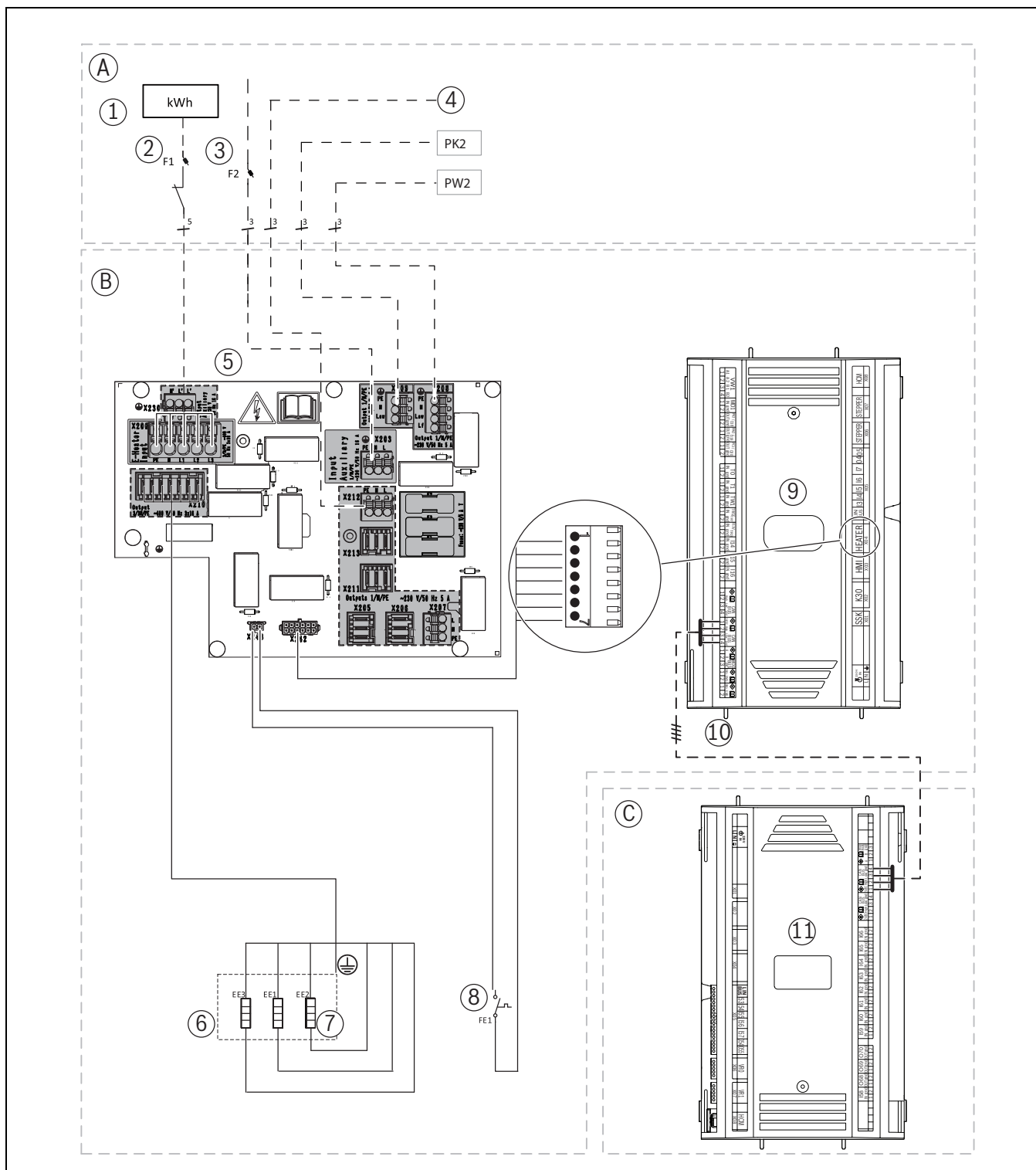
Bild 55 Spannungsversorgung Inneneinheit
