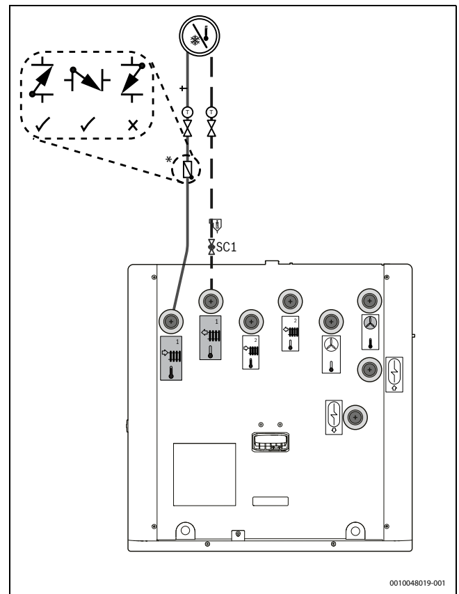
Bild 19 Anschluss der Heizungsanlage
