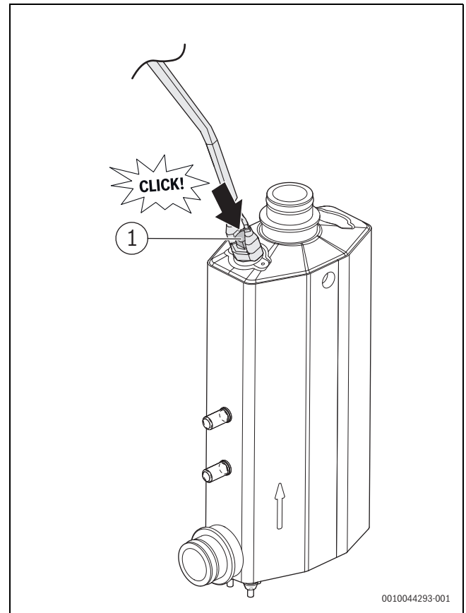
Bild 49 Elektrischer Zuheizer
