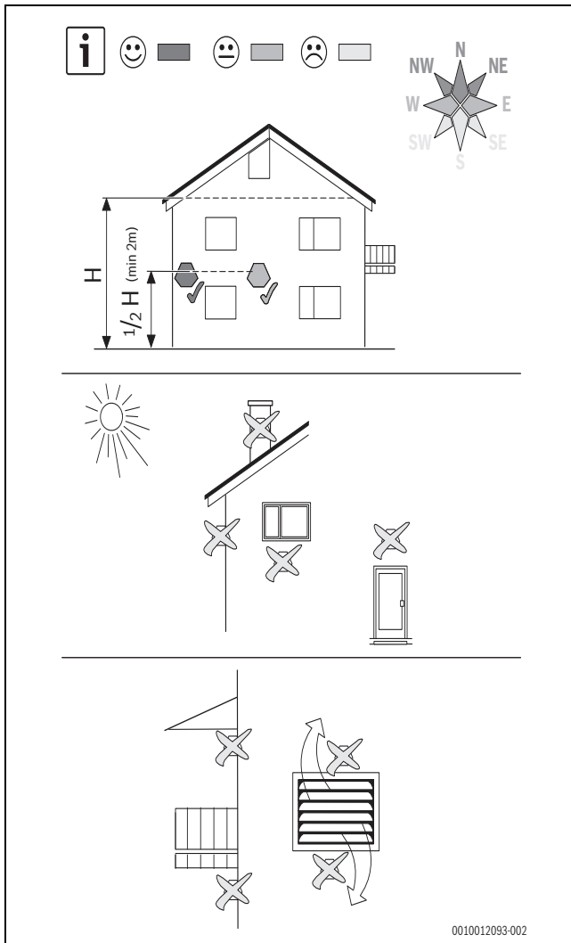
Bild 42 Position des Außentemperaturfühlers
