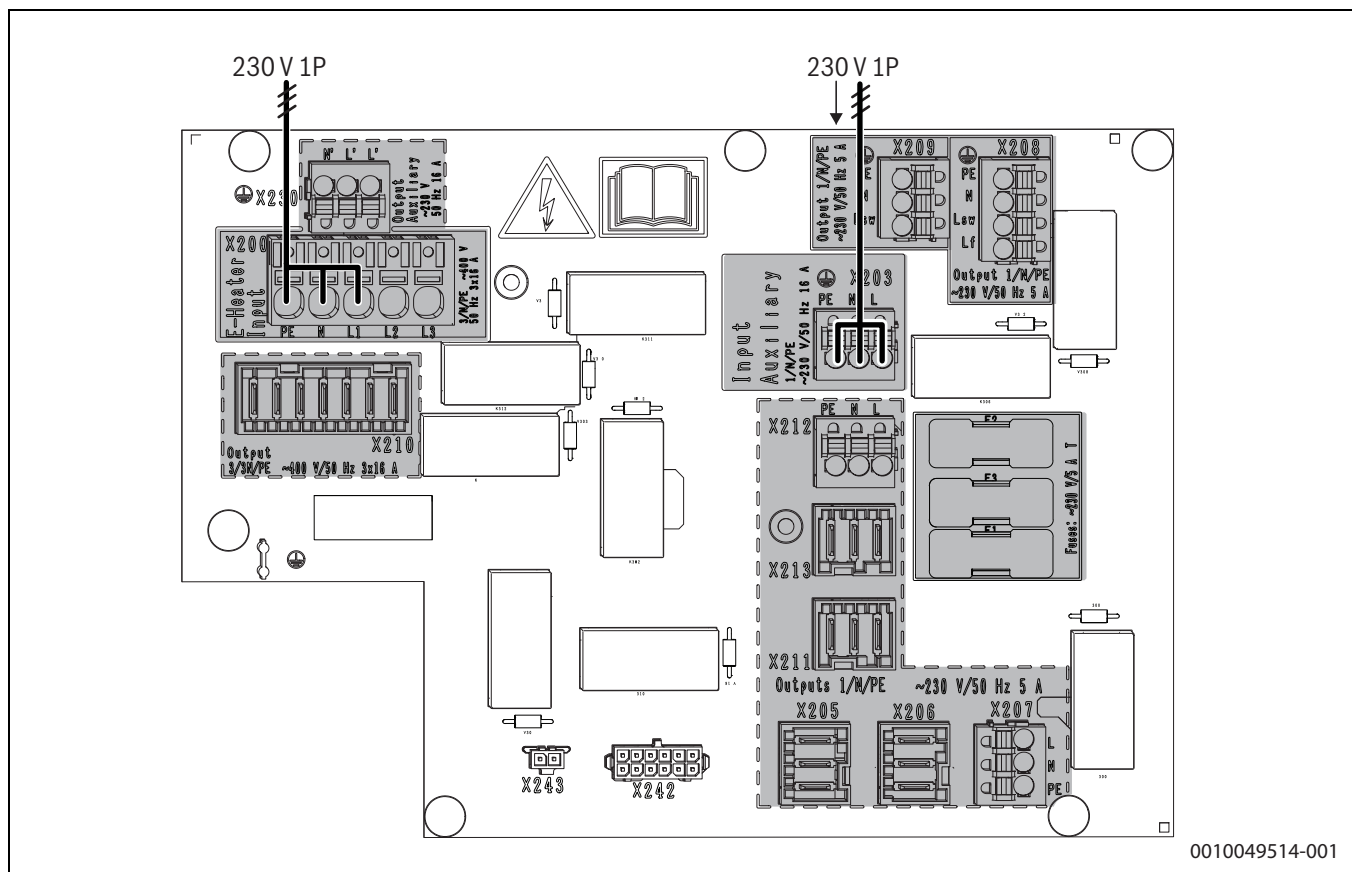
Bild 33 230 V Anschluss für den elektrischen Zuheizer, 230 V Anschluss für Steuerung und Pumpen
