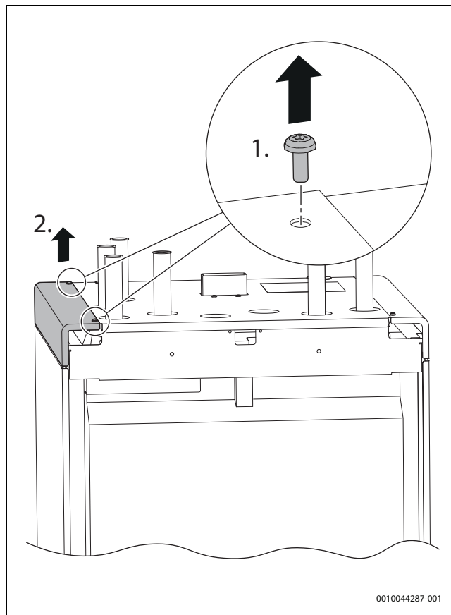
Bild 26 Rückansicht: Ecken mit Befestigungsschrauben
