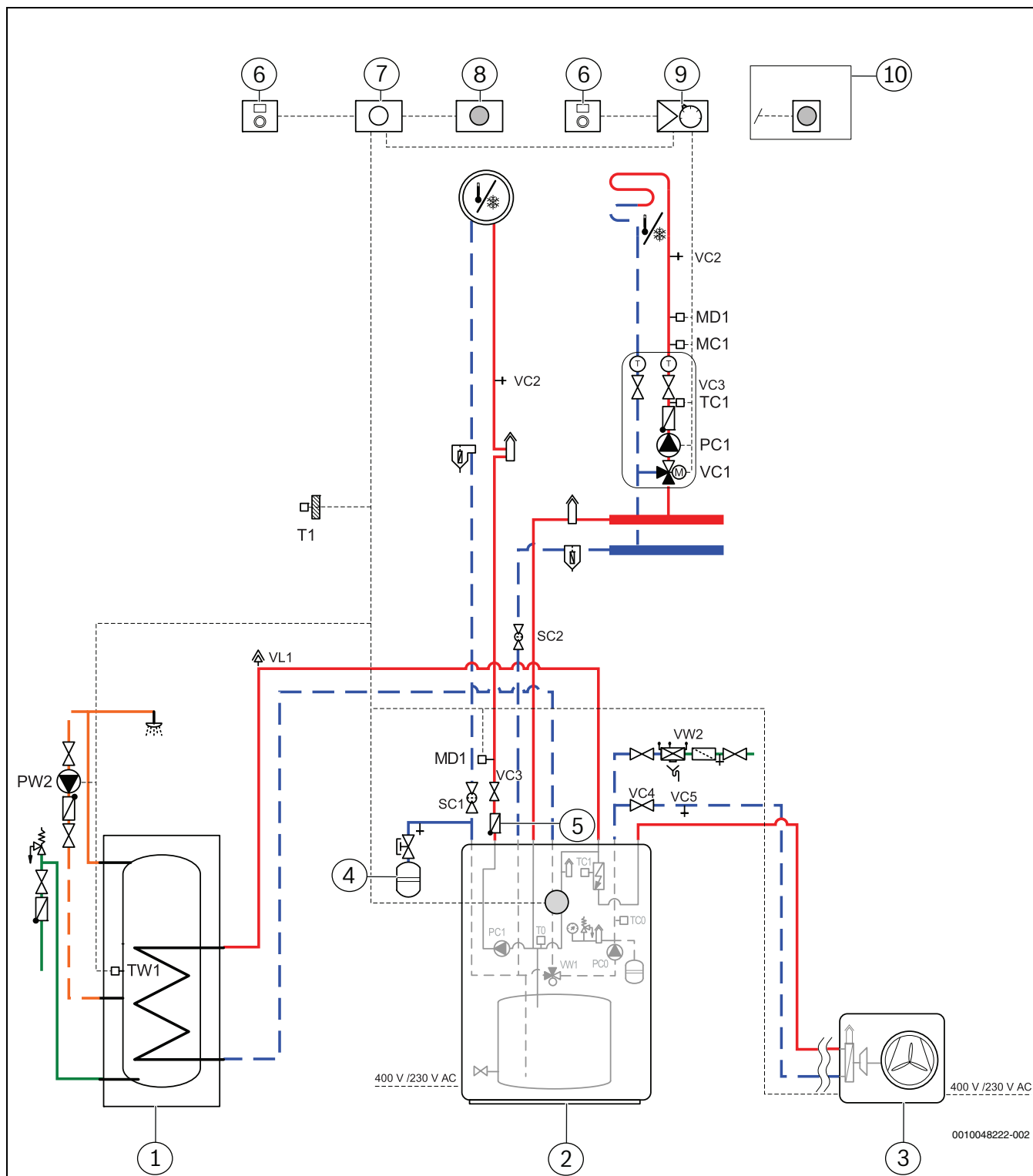
Bild 61 Anlage mit Außeneinheit, Inneneinheit mit integriertem Zuheizer und Pufferspeicher, einem ungemischten und einem gemischten Heizkreis
