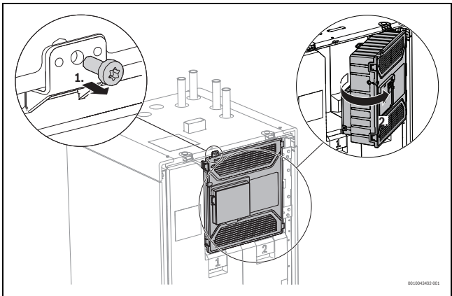
Bild 50 Elektronikbox
