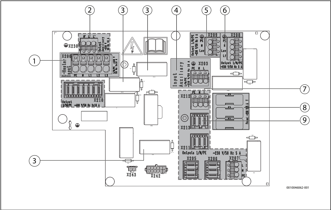
Bild 37 Anschlüsse an der Leiterplatte
