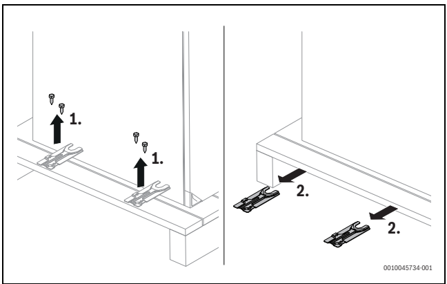
Bild 8 Transportsicherungen entfernen
