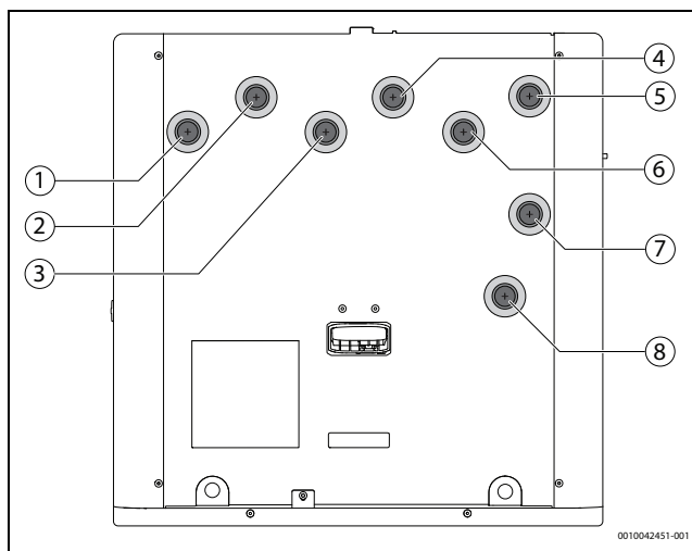
Bild 16 Hydraulische Anschlüsse
