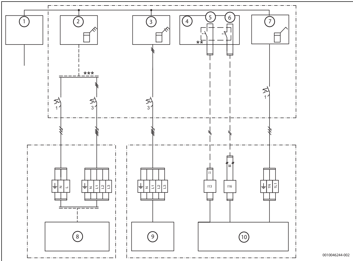
Bild 46 Empfohlene Lösung
