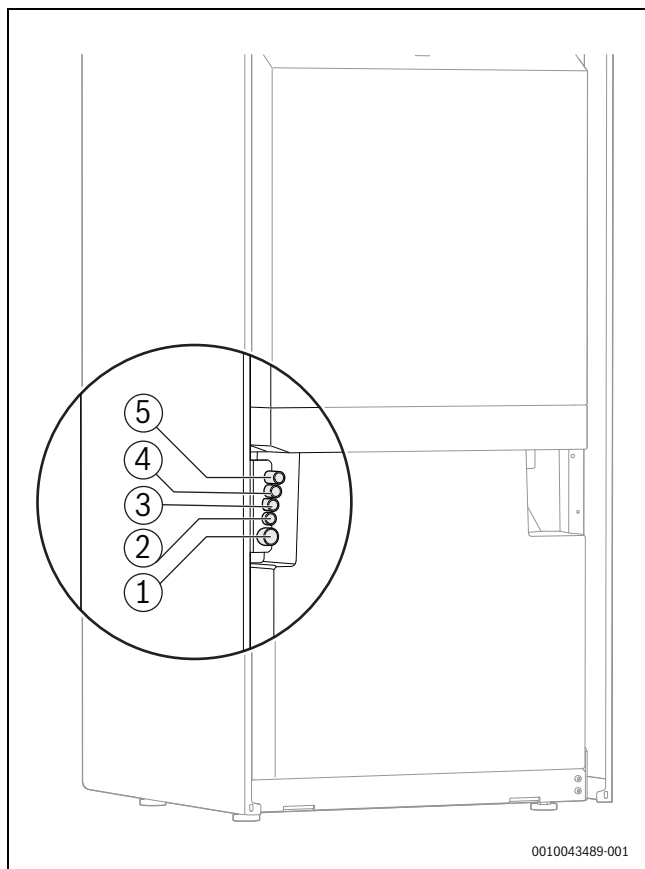
Bild 25 Rückansicht: Kabelführung der Netzkabel in der Inneneinheit
