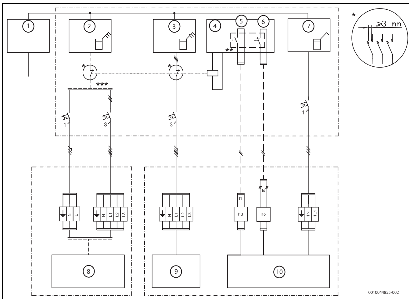
Bild 47 Alternative Lösung
