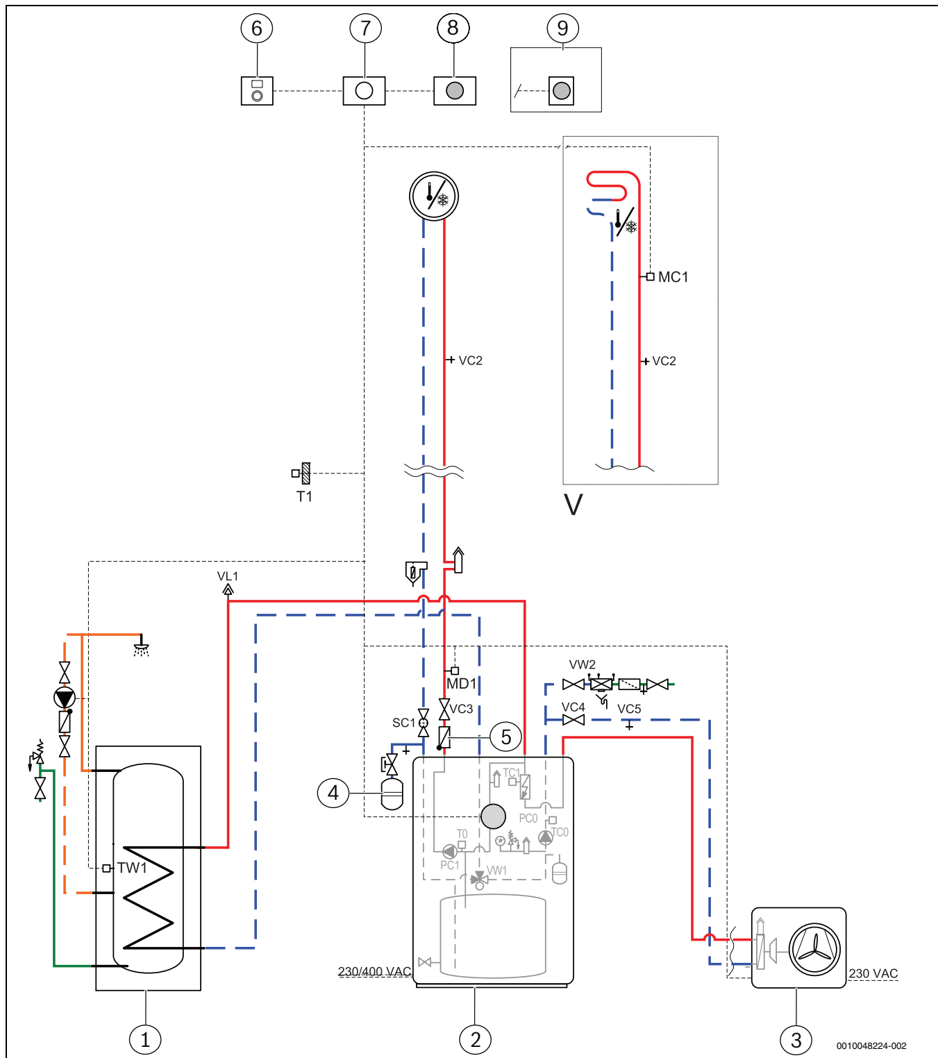
Bild 60 Anlage mit Außeneinheit, Inneneinheit mit integriertem Zuheizter, Pufferspeicher und einem ungemischten Heizkreis
