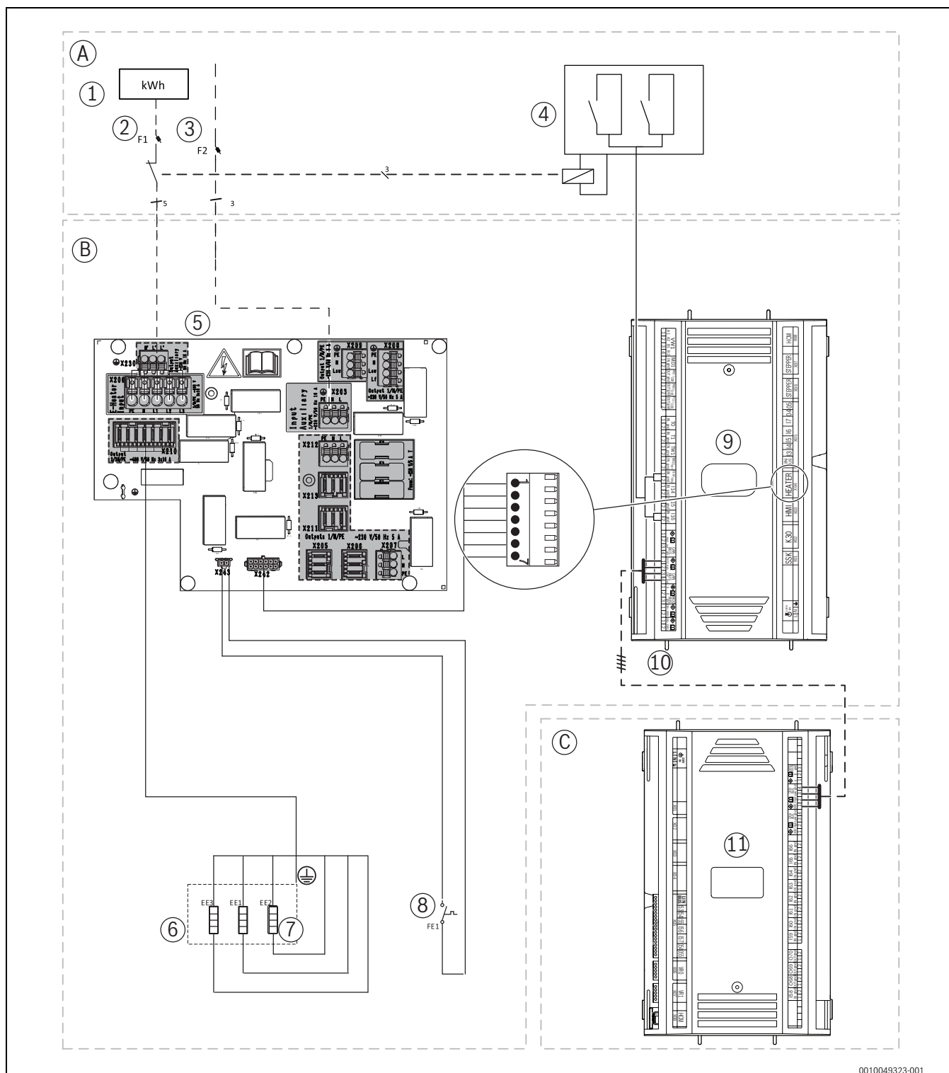
Bild 56 Spannungsversorgung Inneneinheit
