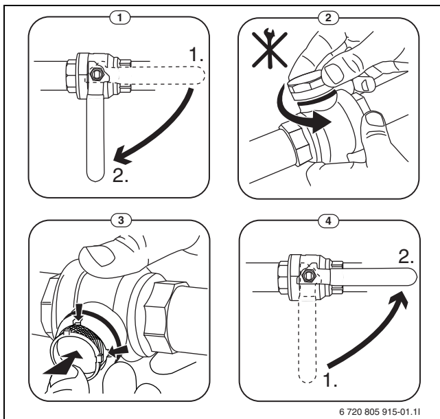
Bild 52 Filterventil reinigen
