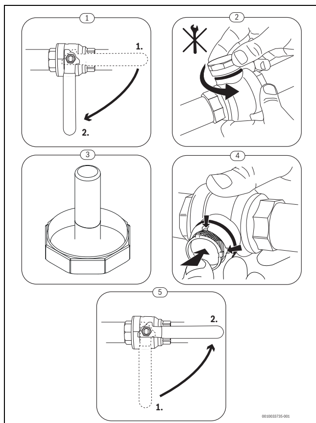
Bild 44 Siebreinigung
