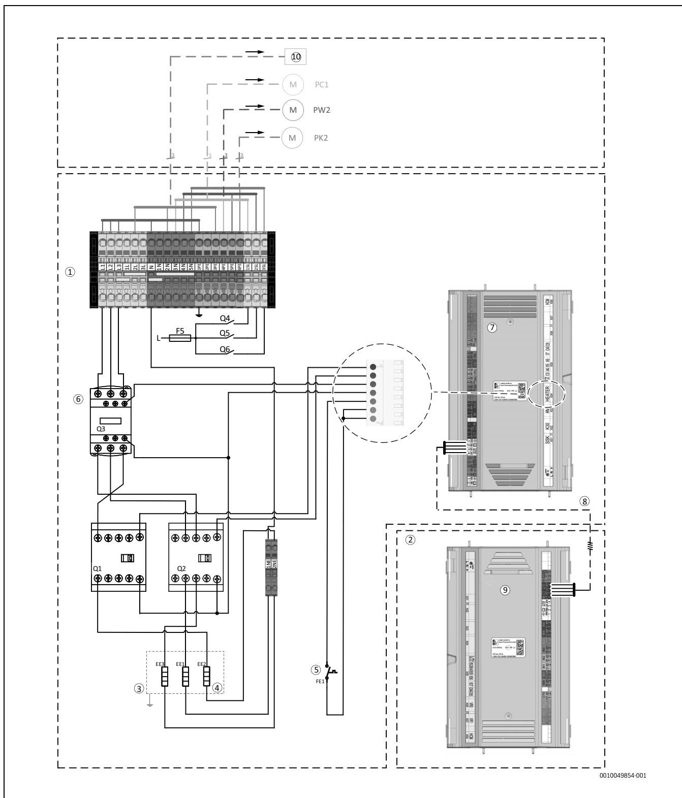
Bild 50 Spannungsversorgung Inneneinheit, Standard
