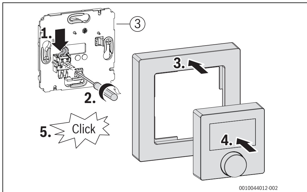
Bild 6 Aufputz-Installation
