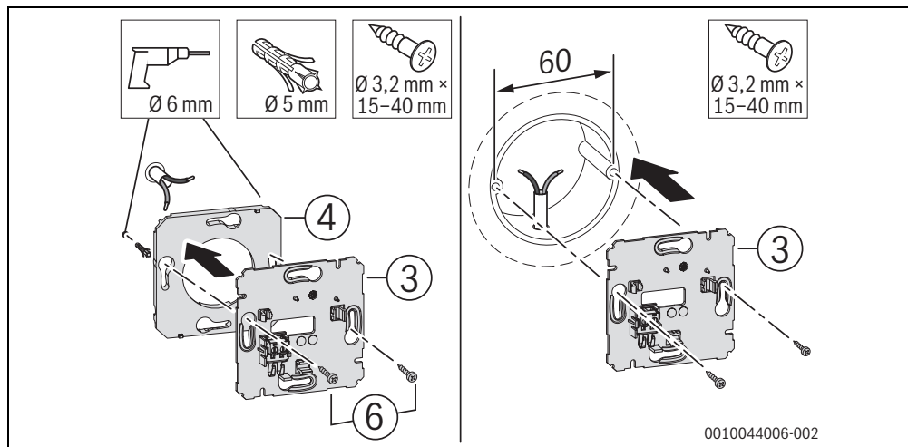
Bild 5 Aufputz-Installation
