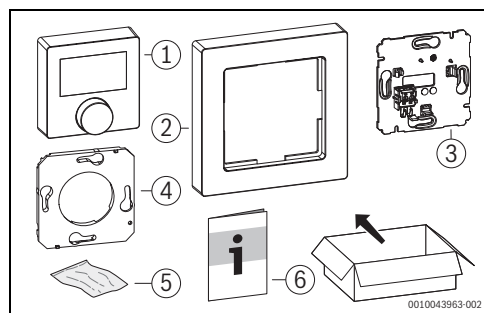
Bild 1 Lieferumfang
