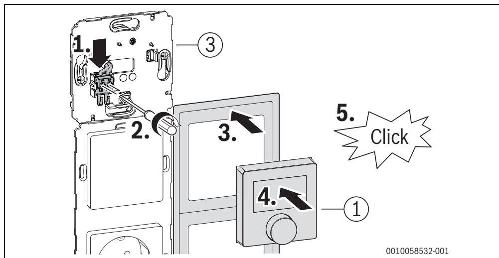
Bild 7 Installation im Lichtschalter mit bauseitigem Rahmen
