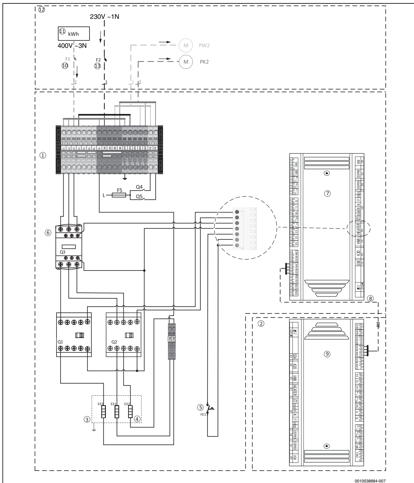
Bild 50 Spannungsversorgung Inneneinheit
