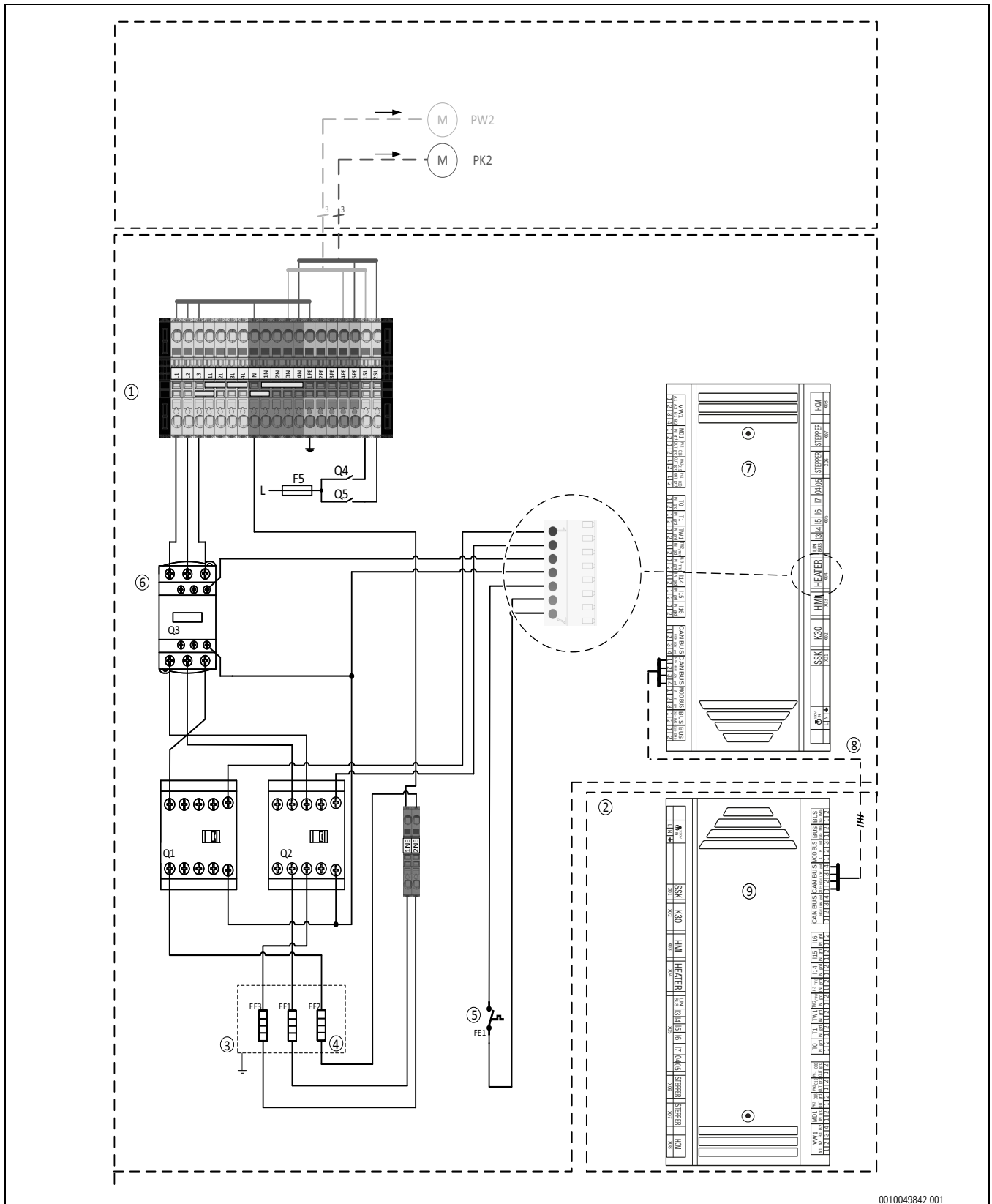
Bild 51 Spannungsversorgung Inneneinheit
