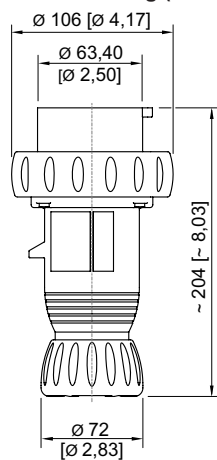
Stecker 3 P + N + PE
