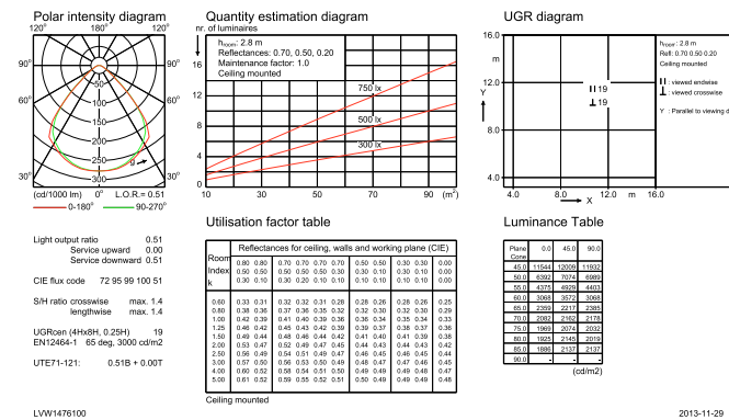
TCS640 2xTL5-54W HFP AC-MLO
