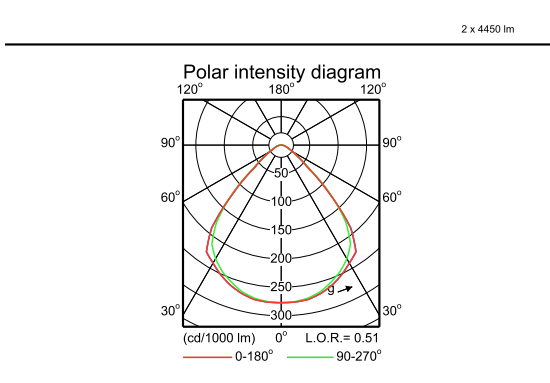
TCS640 2xTL5-54W HFP AC-MLO
