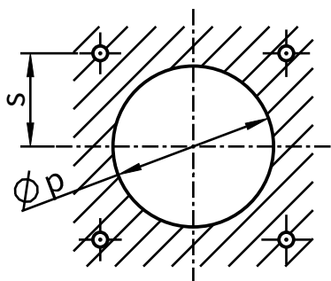
Montageausschnitt/ Mounting cutout
