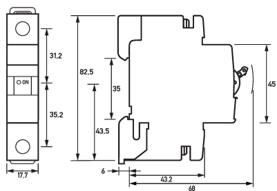
Maßzeichnung Leitungsschutzschalter DLS 6i B20-1
