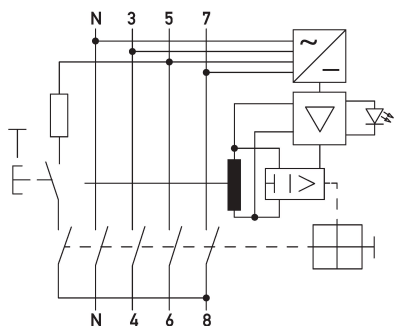
Schaltungsbeispiel Fehlerstromschutzschalter DFS 4 063-4/0,10-PV
