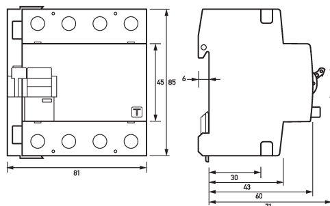
Maßzeichnung Fehlerstromschutzschalter DFS 4 100-4/0,03-B SK NA
