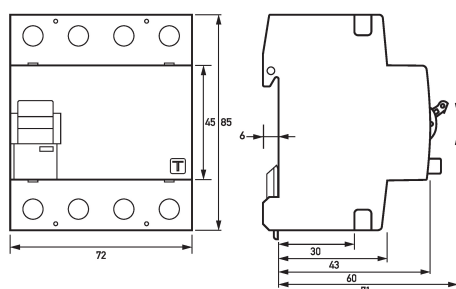
Maßzeichnung Fehlerstromschutzschalter DFS 4 040-4/0,30-A R
