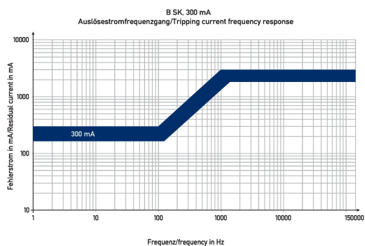
Diagramme Fehlerstromschutzschalter DFS 4 063-4/0,30-B SK NA
