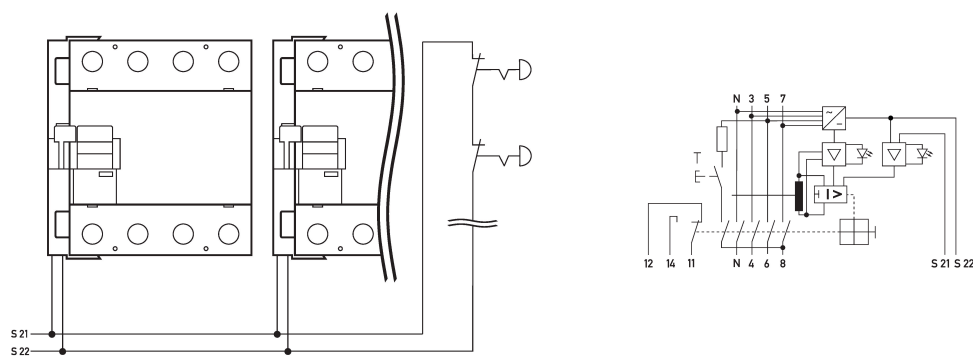
Schaltungsbeispiel Fehlerstromschutzschalter DFS 4 063-4/0,30-B SK NA
