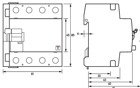
Maßzeichnung Fehlerstromschutzschalter DFS 4 063-4/0,30-B SK NA
