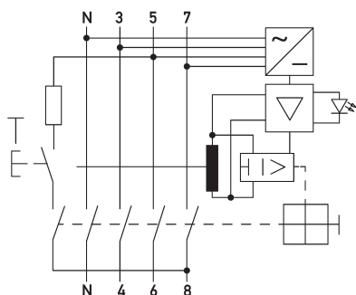
Schaltungsbeispiel Fehlerstromschutzschalter DFS 4 063-4/0,30-B SK ISO HD
