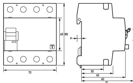
Maßzeichnung Fehlerstromschutzschalter DFS 4 063-4/0,50-B SK ISO HD
