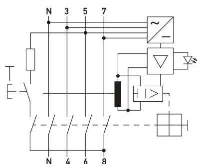
Schaltungsbeispiel Fehlerstromschutzschalter DFS 4 063-4/0,50-B SK ISO HD
