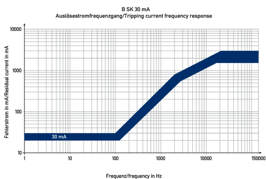
Diagramme Fehlerstromschutzschalter DFS 4 040-4/0,03-B SK R HD
