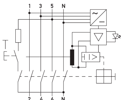
Schaltungsbeispiel Fehlerstromschutzschalter DFS 4 040-4/0,03-B SK R HD
