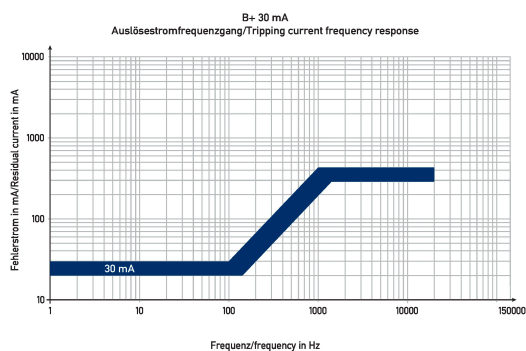
Diagramme Fehlerstromschutzschalter DFS 4 125-2/0,03-B+
