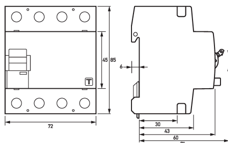
Maßzeichnung Fehlerstromschutzschalter DFS 4 125-4/0,03-A V500
