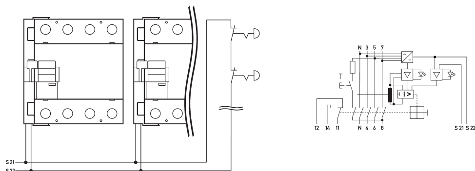
Schaltungsbeispiel Fehlerstromschutzschalter DFS 4 125-4/0,03-B SK NA
