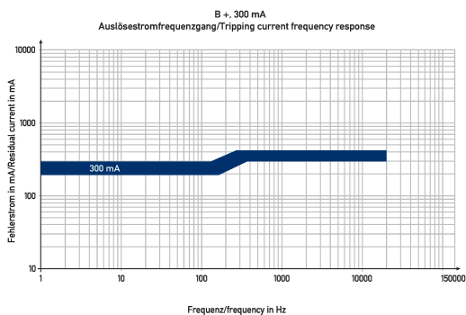
Diagramme Fehlerstromschutzschalter DFS 4 125-4/0,30-B+ HD
