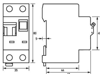
Maßzeichnung FI-/LS-Kombinationen DRCBO 3 B20/0,03/1N-A
