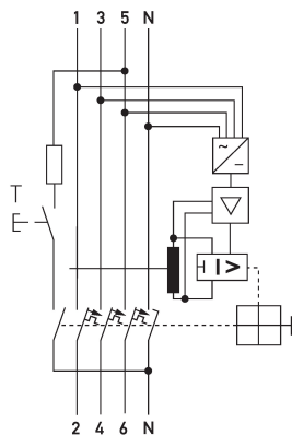
Schaltungsbeispiel FI-/LS-Kombinationen DRCBO 4 C20/0,03/3N-B SK
