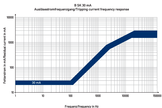
Diagramme FI-/LS-Kombinationen DRCBO 4 C20/0,03/3N-B SK
