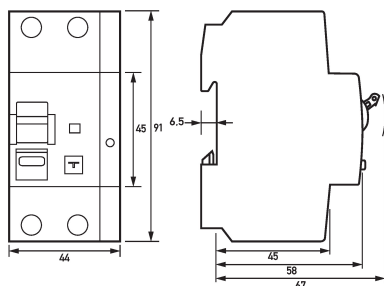
Maßzeichnung FI-/LS-Kombinationen DRCBO 4 Bo6/o,03/1N-B NK
