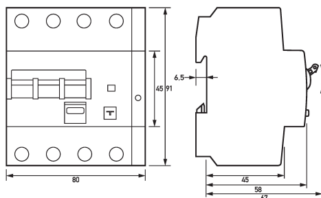
Maßzeichnung FI-/LS-Kombinationen DRCBO 4 C32/0,30/3N-B+
