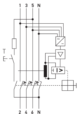
Schaltungsbeispiel FI-/LS-Kombinationen DRCBO 4 B16/o,30/3N-B NK
