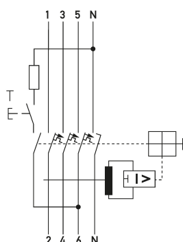
Schaltungsbeispiel FI-/LS-Kombinationen DRCBO 4 C10/0,03/3N-A
