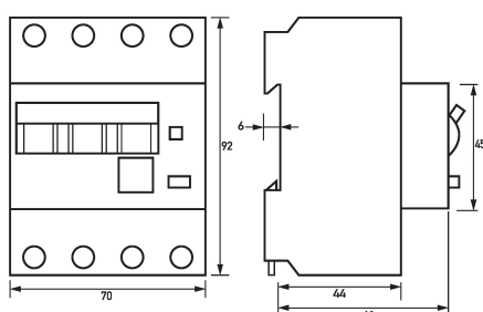
Maßzeichnung FI-/LS-Kombinationen DRCBO 4 C10/0,03/3N-A
