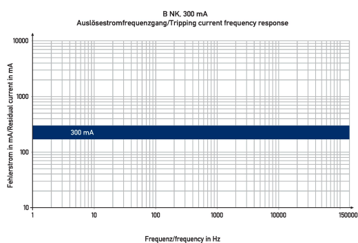
Diagramme FI-/LS-Kombinationen DRCBO 4 C25/0,30/3N-B NK
