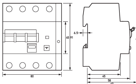
Maßzeichnung FI-/LS-Kombinationen DRCBO 4 C32/0,03/3N-B+
