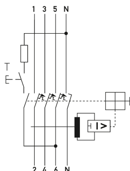
Schaltungsbeispiel FI-/LS-Kombinationen DRCBO 4 C16/0,30/3N-A
