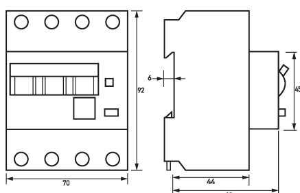
Maßzeichnung FI-/LS-Kombinationen DRCBO 4 C16/0,30/3N-A
