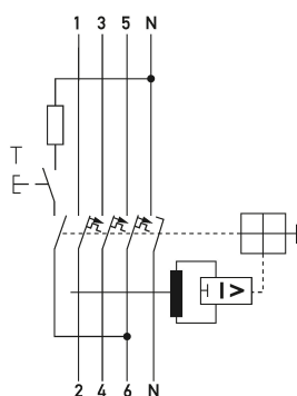
Schaltungsbeispiel FI-/LS-Kombinationen DRCBO 4 B10/0,03/3N-A
