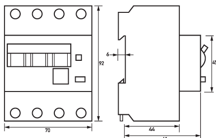
Maßzeichnung FI-/LS-Kombinationen DRCBO 4 B10/0,03/3N-A
