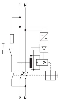
Schaltungsbeispiel FI-/LS-Kombinationen DRCBO 4 C20/0,03/1N-B NK
